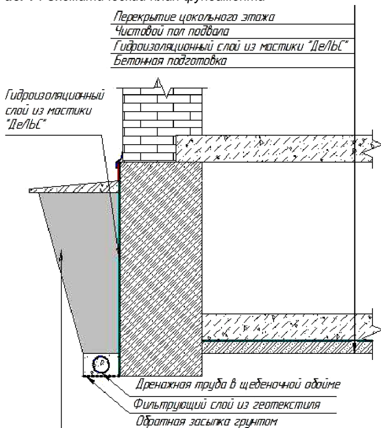
Рис. 1 : Схематический план фундамента
